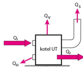
Tepelné ztráty kotle na tuhá paliva
