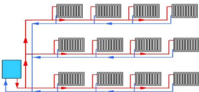
Princip ústředního vytápění
