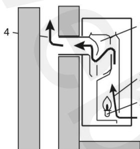
Plynové lokální topidlo otevřené konstrukce
