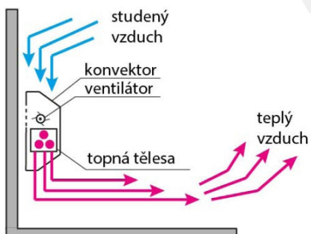
Elektrický konvektor
