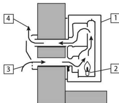
Plynové lokální topidlo uzavřené konstrukce
