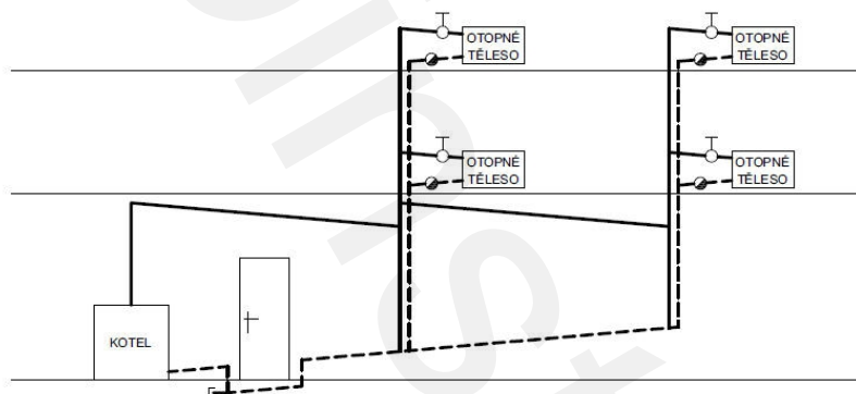
Parní otopná soustava se spodním rozvodem
