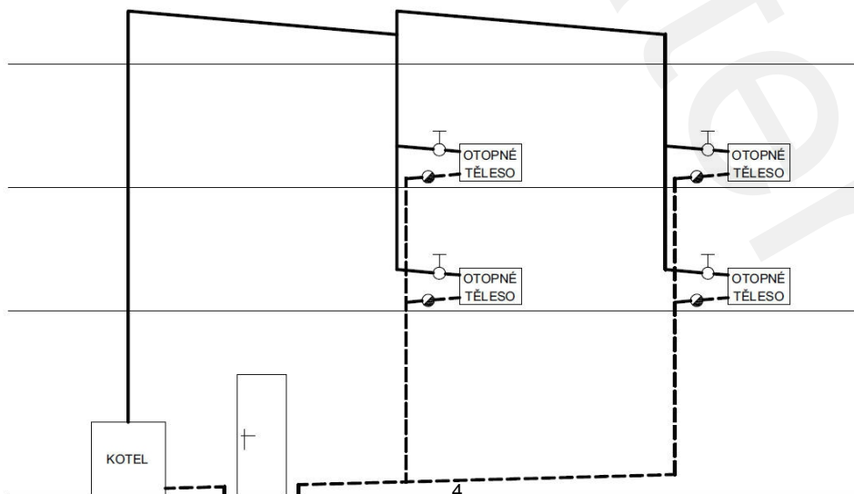
Parní otopná soustava s horním rozvodem
